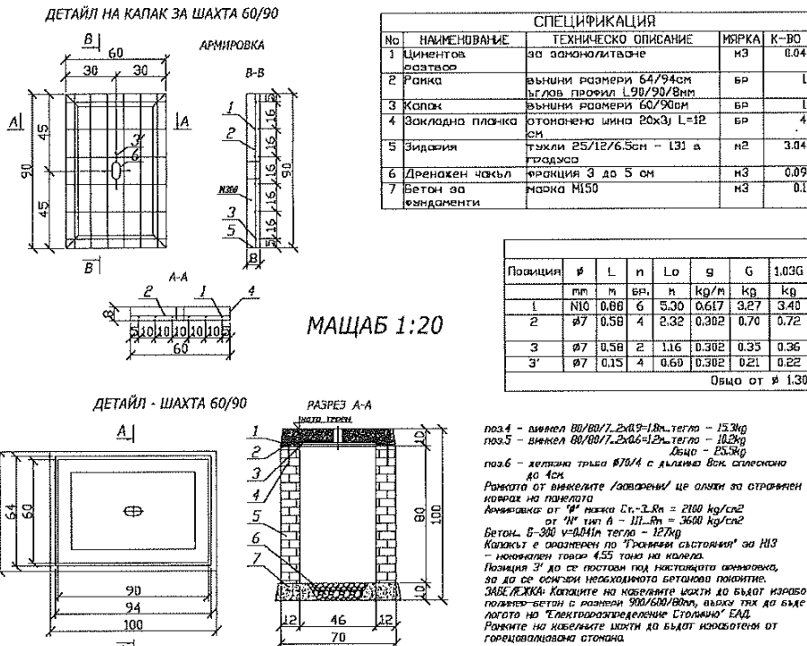
Фиг.6.3. Кабелна шахта – единична
